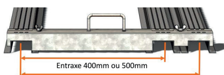
Gabarit platelage bois et composite
